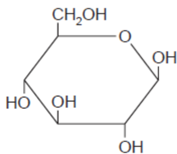
molecule Y
